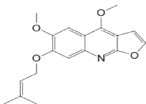
Pteleine (6)
