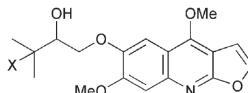
chlorodesnkolbisine (5), X=Cl
