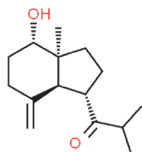
Teclenone A (25)
