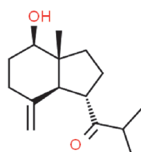
Teclenone B (26)
