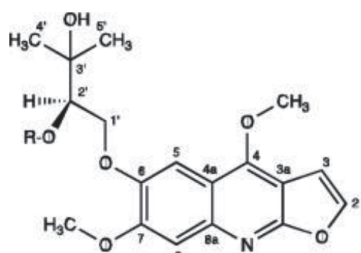
Montrifoline ( R=H) (14)
