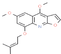
Tectelebine (1)
