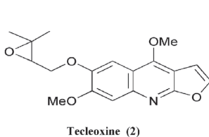
Tecteleoxine (2)
