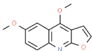
Nobiline (8)
